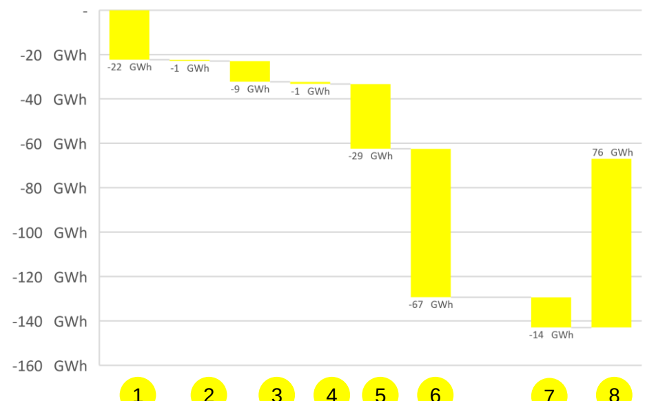
Potentiel de réduction des consommations d'énergie - Secteur Transports
