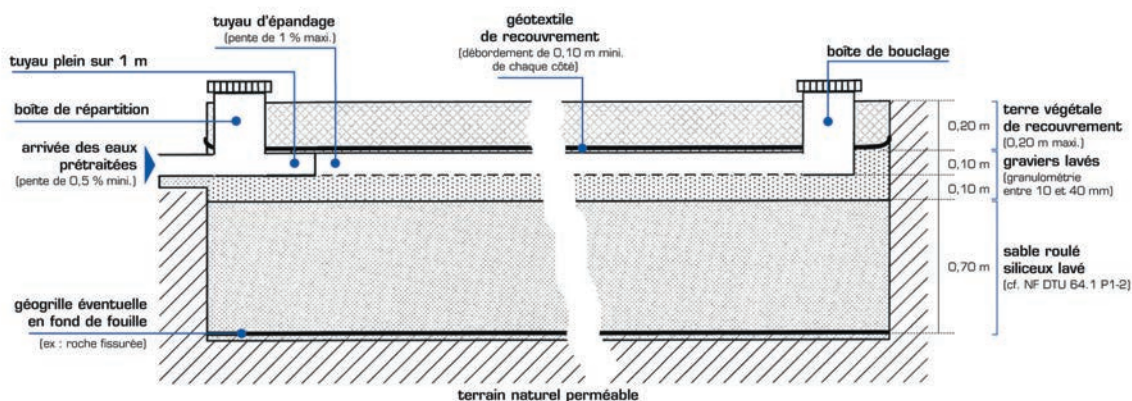
coupe longitudinale
